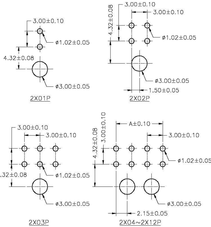
P.C.B LAYOUT
