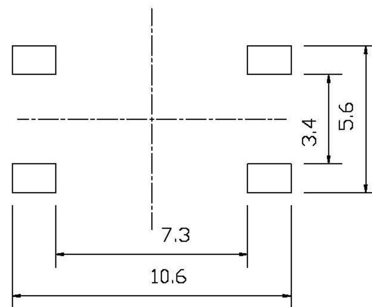
印制线路板(PCB Layout)
