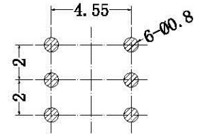
PCB参考图
